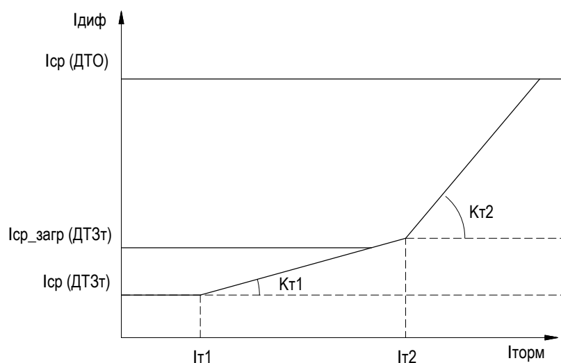
Рисунок 2.1 – Характеристика срабатывания ДТЗТ
